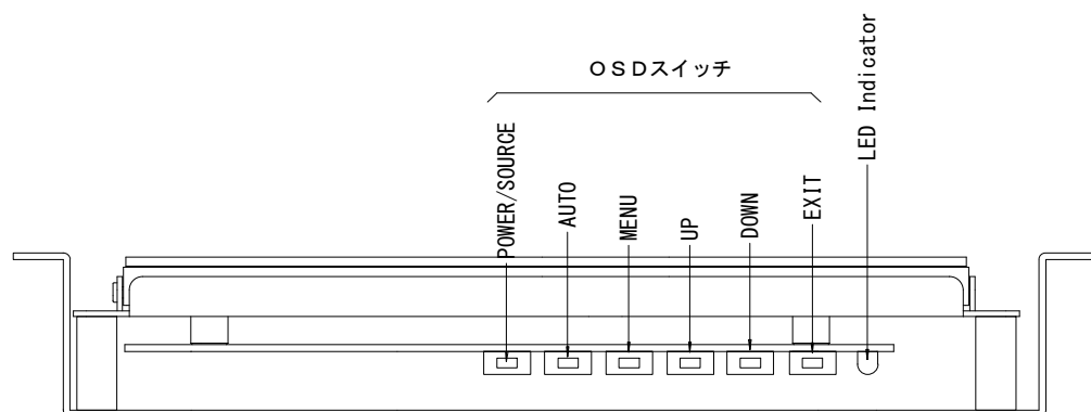
背面図
