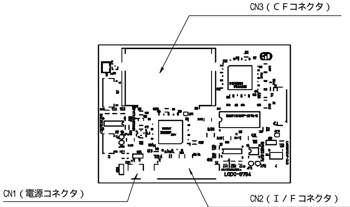
制御基板背面図
