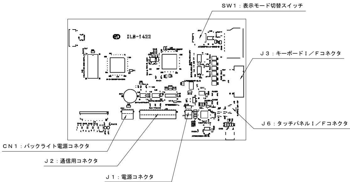
制御基板背面図
